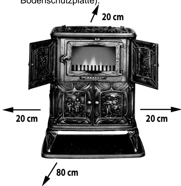
Abbildung 4: Sicherheitsabstände
