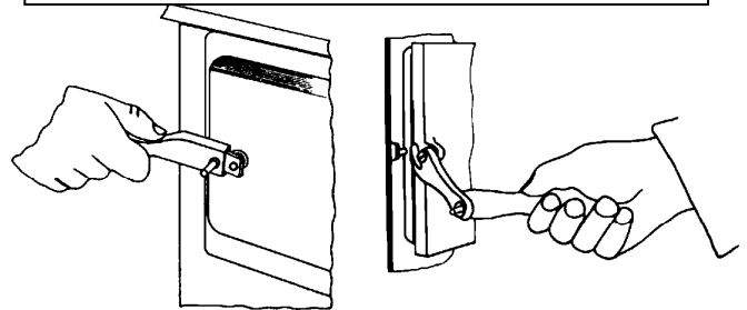
Abbildung 11: Bedienung des Rüttelhebels
