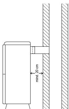
Abbildung 1: direkter Anschluß, Abstand zur Stellwand
